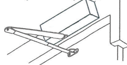
3. Top Jamb Mount (Push Side)
