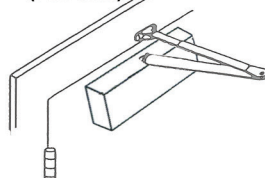
2. Standard Mount (Pull Side)
